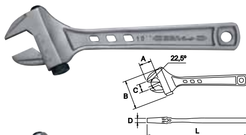
Llave ajustable con moleta lateral Adjustable wrench with lateral turning knob Clé à molette avec molette latérale
